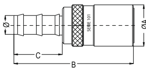
Push lock hose tail coupler Kupplung mit Schnellsteck - Schlauchtülle
