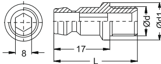
Plug with valve (059 serie) Verschlussnippel ( 059 serie )
