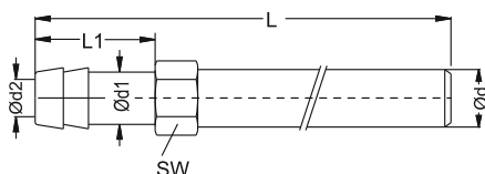
Hose tail extension Schlauchtülle Verlängerung
