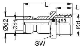
Plug with valve ( 090 serie ) Verschlussnippel ( 090 serie )
