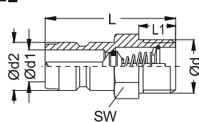
Plug with valve ( 190 serie ) Verschlussnippel ( 190 serie )
