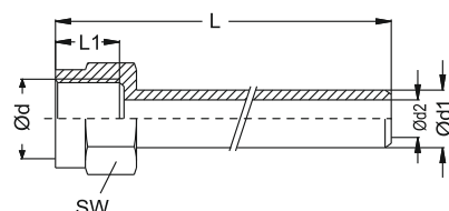
Sealing plug extension / Dichtungsnippel mit Verlängerung
