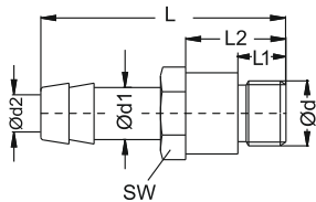
Hose nipple / Nippel mit Schlauchtülle
