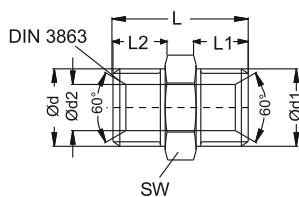
Double nipples / Doppelnippel
