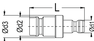
Adapting Plug 060 - 090 Adapternippel 060 - 090
