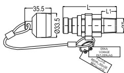
NPT Male Threaded shut-off Plug Verschlussnippel mit NPT Aussengewinde
