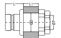
Built-in Plug Verschlussnippel mit Schottverschraubung
