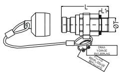
Male Threaded shut-off Plug Verschlussnippel mit Aussengewinde
